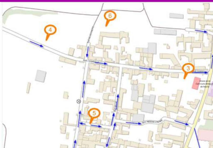
Figure 7 : Caractérisation des écoulements et localisation des pistes d'action de réduction des effets
